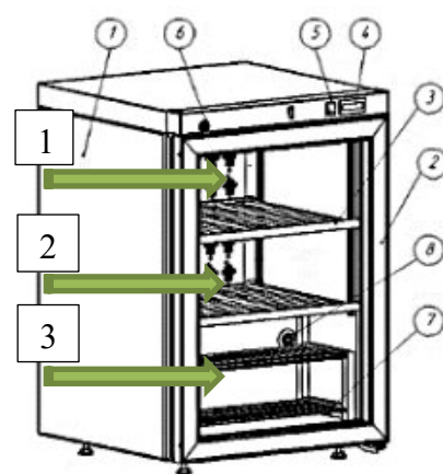
Рис.2. Внешний вид шкафа DW102-Bravo.
