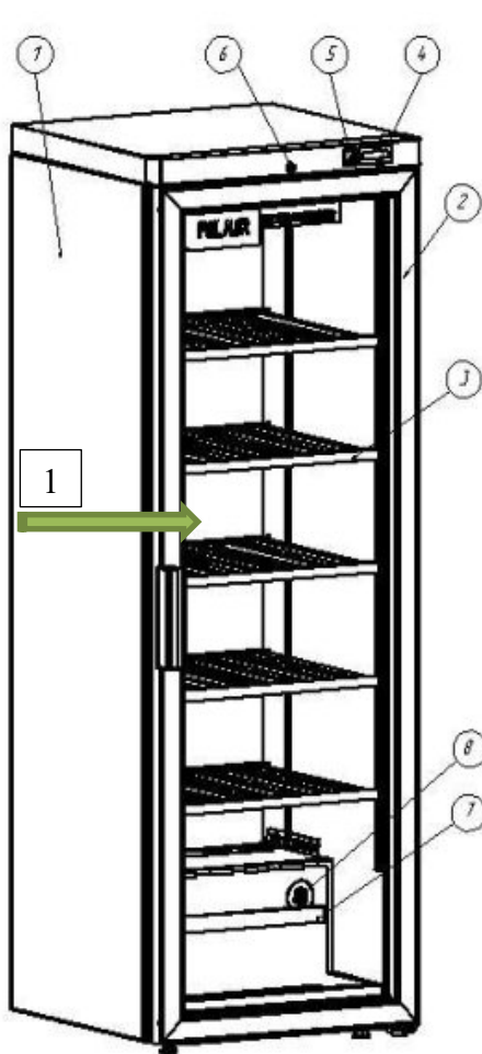
Рис.3. Внешний вид шкафа DW104u-Bravo.
