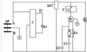
SD-516AELC/AEL
