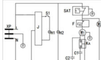
SD-516AMLC/AML
