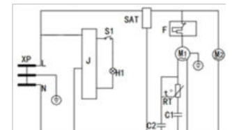
SD-206/336/416AELC/AEL XP - штепсель ашасы; SAT - Термостат; S1 - артқы жарық қосқышы; F - қорғаныс релесі; J - қуат қалқаны; M1 - Компрессор; H1 - ішкі подстветка; M2 - желдеткіш салқындату; RT - Стартер; C1 - іске қосу сыйымдылығы (жүзеге асыру кезінде); C2 - пайдалану сыйымдылығы (жүзеге асыру кезінде)
