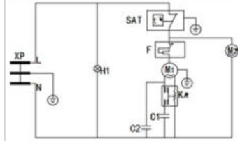
SD-516AMC/AM XP - штепсель ашасы; SAT - Термостат; F - қорғаныс релесі; H1 - қуат индикаторы; M1 - Компрессор; M2 - желдеткіш салқындату; KA - Стартер; C1 - іске қосу сыйымдылығы (жүзеге асыру кезінде); C2 - пайдалану сыйымдылығы (жүзеге асыру кезінде)
