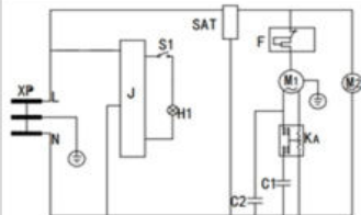
SD-516AELC/AEL
