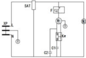
SD-516AEC/AE XP - Штепсельді айыр; SAT- Термостат; F – Қорғаныс релесі; M1-Компрессор; M2 - салқындату желдеткіші; KA-Стартер C1 - іске қосу сыйымдылығы (жүзеге асыру кезінде); C2 - пайдалану сыйымдылығы (жүзеге асыру кезінде)
