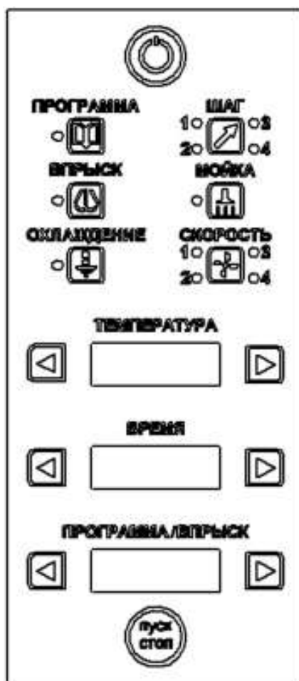
Рис. 3. Внешний вид панели управления КЭП-6П-01 и КЭП-10П-01
