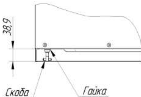
Рис. 7. Регулировка замкового устройства
