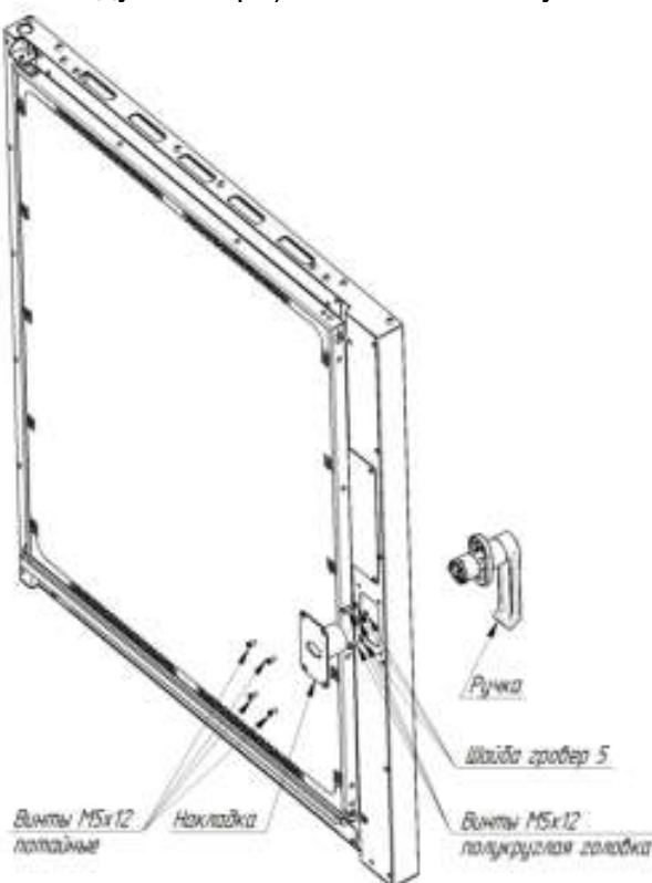
Рис. 4. Замена ручки
