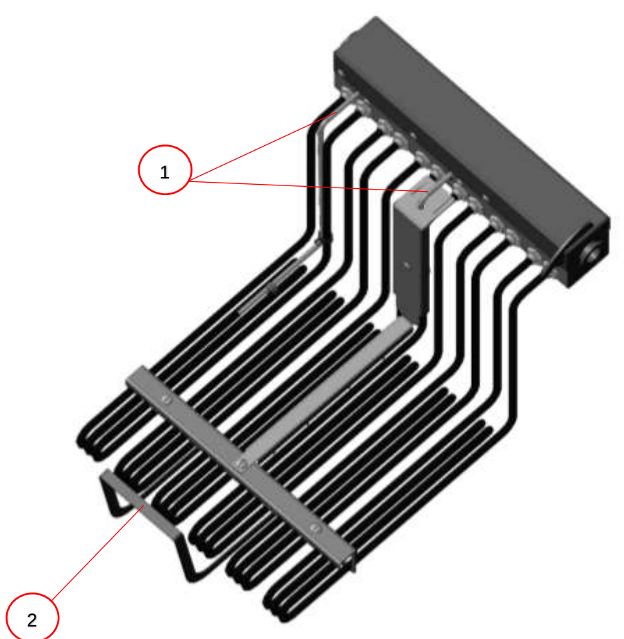
Рисунок 2 – ТЭНы. 1 – Термостат (2 шт.); 2 – Ручка.
