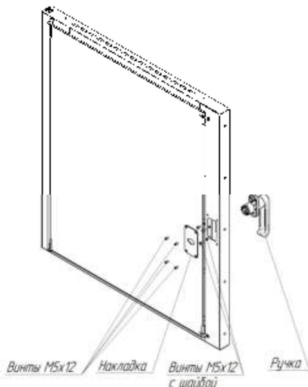
Рис. 6. Замена ручки
