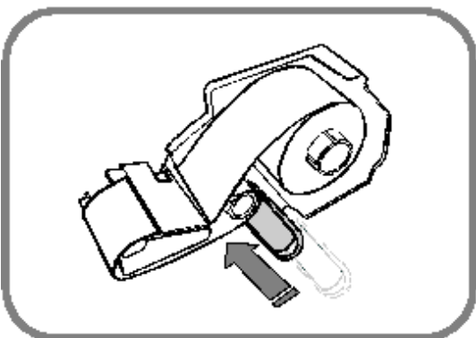
Рисунок 1.15 – Фиксация ленты на приёмной катушке
