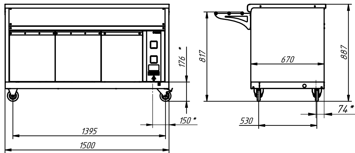
Вариант с поворотными колесами
