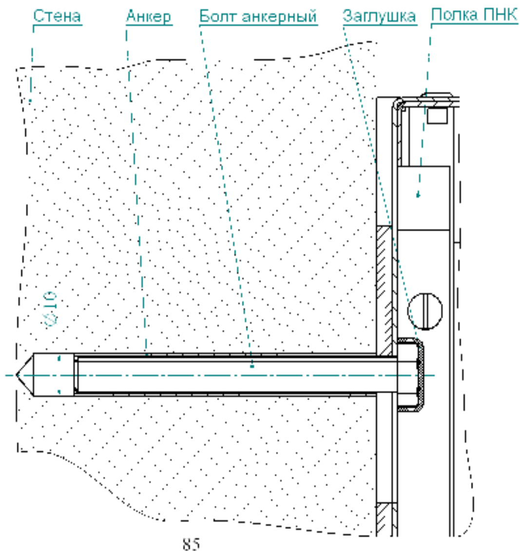
Рисунок 1. Пример крепления полки ПНК.
