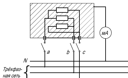
Рисунок 4 — Схема измерения тока утечки
