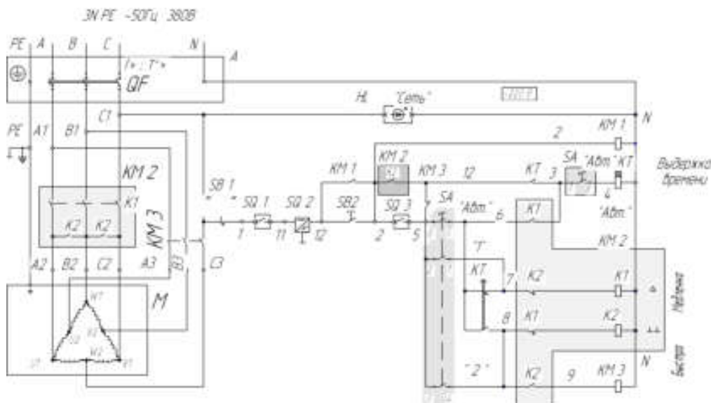
A—устройство ввода; HL—арматура светосигнальная; KM1...KM3—пускатели; SB1, SB2—кнопки; KT—реле времени; M—электродвигатель; QF—выключатель автоматический; SA—переключатель; SQ1—выключатель путевой (контроль фиксации головной части); SQ2—выключатель путевой (контроль крышки дежи); X1, X2—блоки зажимов; XS1, XS2—клеммы ножевые; XS3...XS6—соединители.
