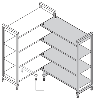
Стойки для нижних крепежных полок
