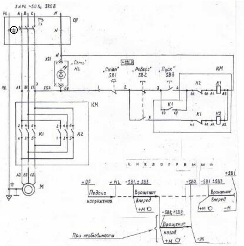
QF - выключатель автоматический; HL - арматура светосигнальная; KM - пускатель; M - электродвигатель; SB1, SB2, SB3 - кнопки; XS1, XS2 - соединители Рисунок 4 - Схема электрическая принципиальная
