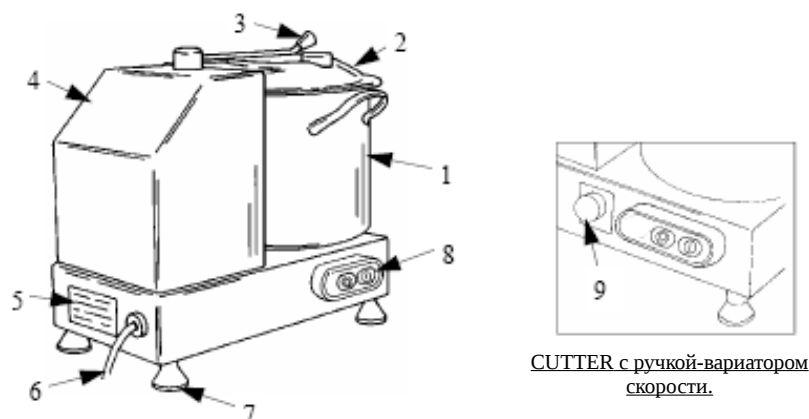
Иллюстрация 1. Общий вид машины
