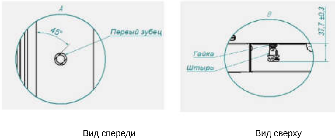
Рис. 4. Регулировка замкового устройства
