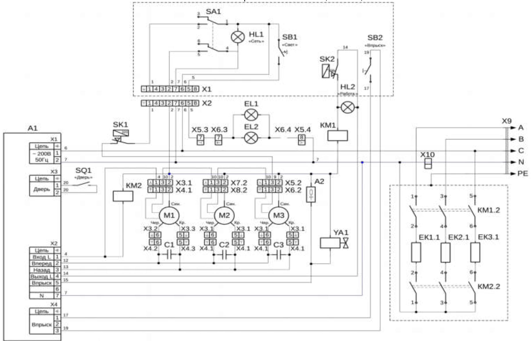
СХЕМА ЭЛЕКТРИЧЕСКАЯ ПРИНЦИПАЛЬНАЯ КЭП-6, КЭП-6Э, КЭП-10 и КЭП-10Э
