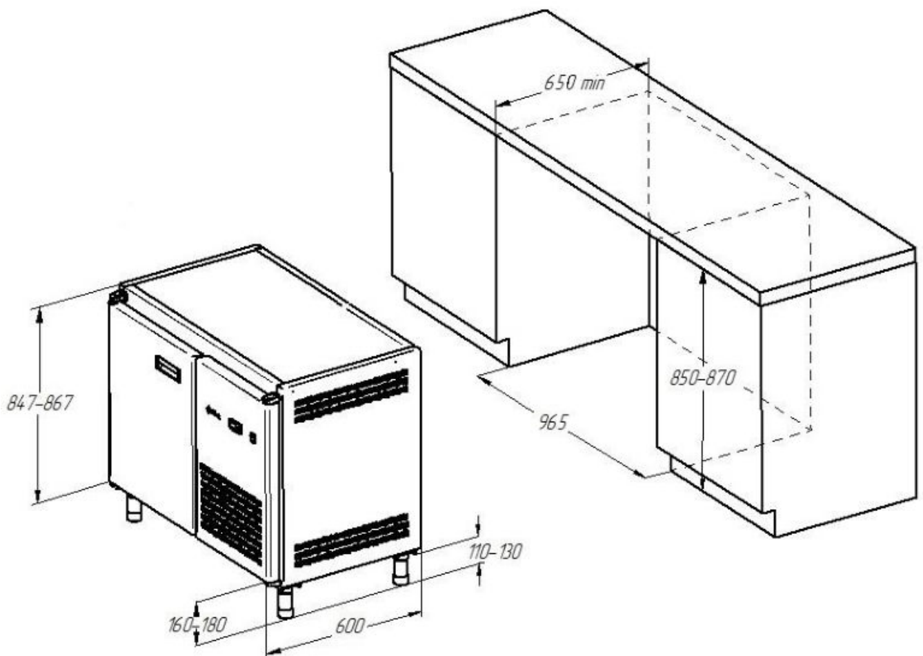
Рис.24. Схема встраивания CXH-60 без столешницы (дверь).
