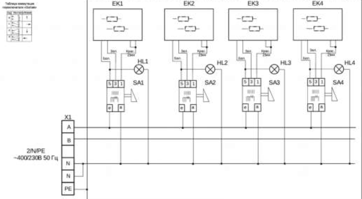
Рис.4 Схема электрическая принципиальная для всех ЭП-4П
